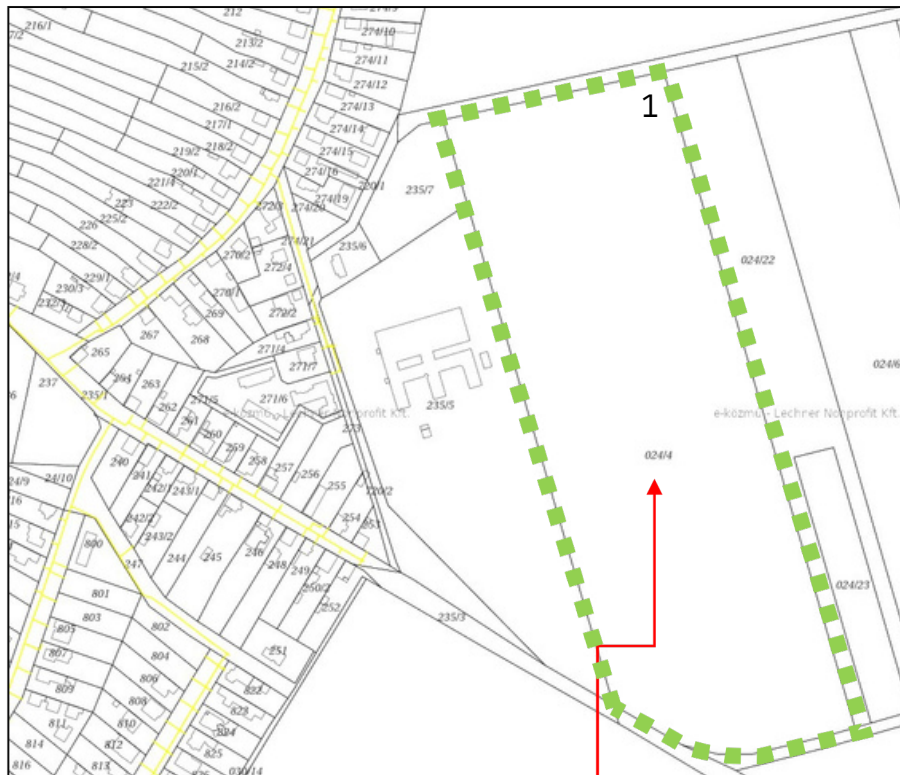
Máriakálnok a feladatleírás 1) pontjában szereplő módosítással érintett terület mai gázenergia hálózata. A módosítással érintett telkek /Forrás: e-közművek/
