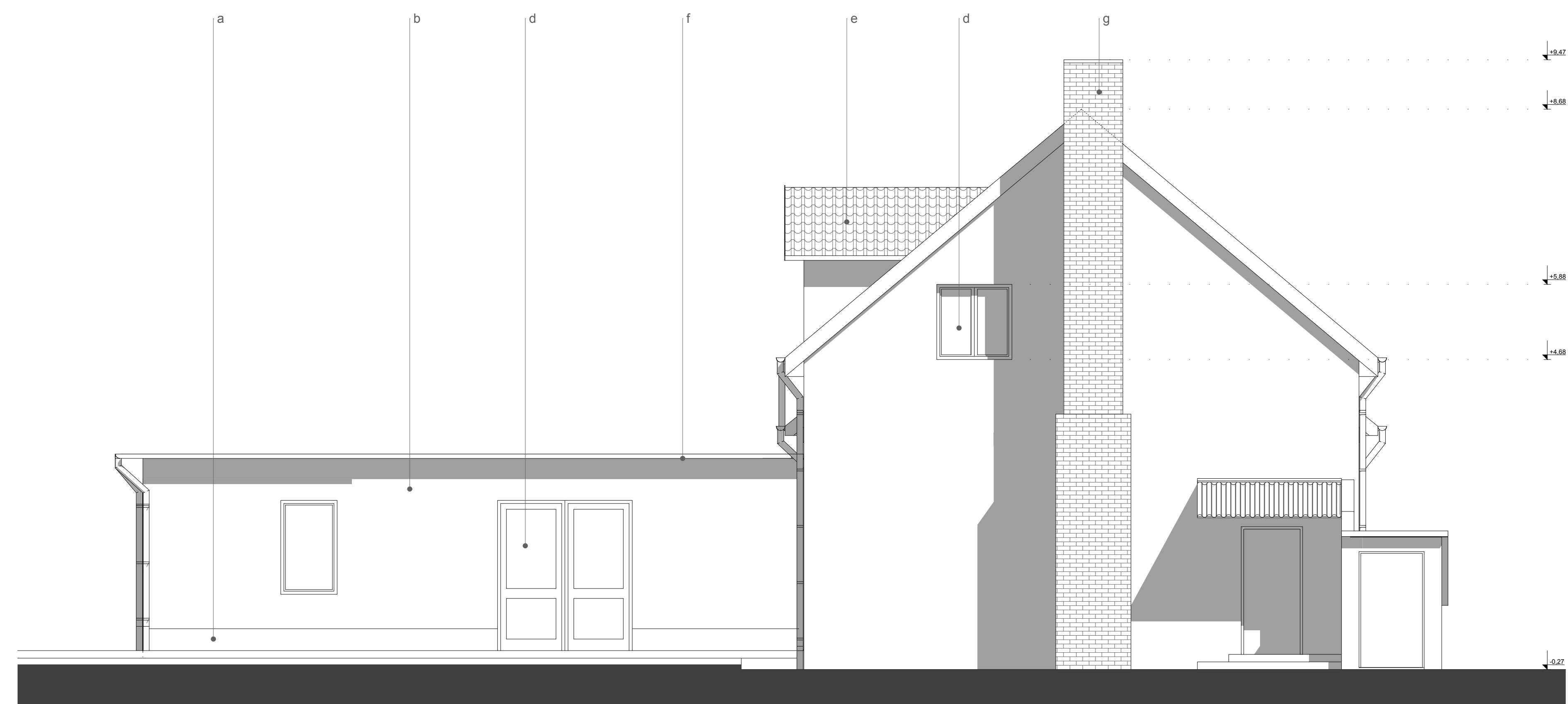
tervezett észak-nyugati homlokzat m 1_50
